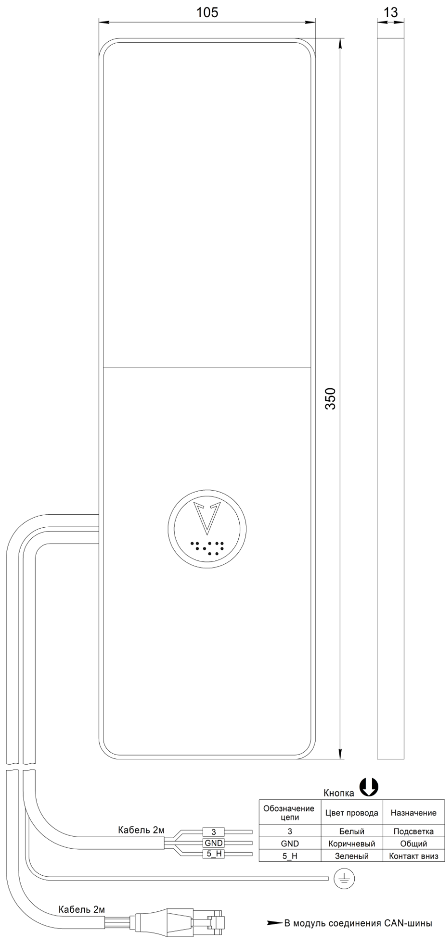
Рис.1 Внешний вид, габаритные и установочные размеры Вызывного поста МАЛАХИТ (жгут RJ45) НШЕК.468381.015-01
